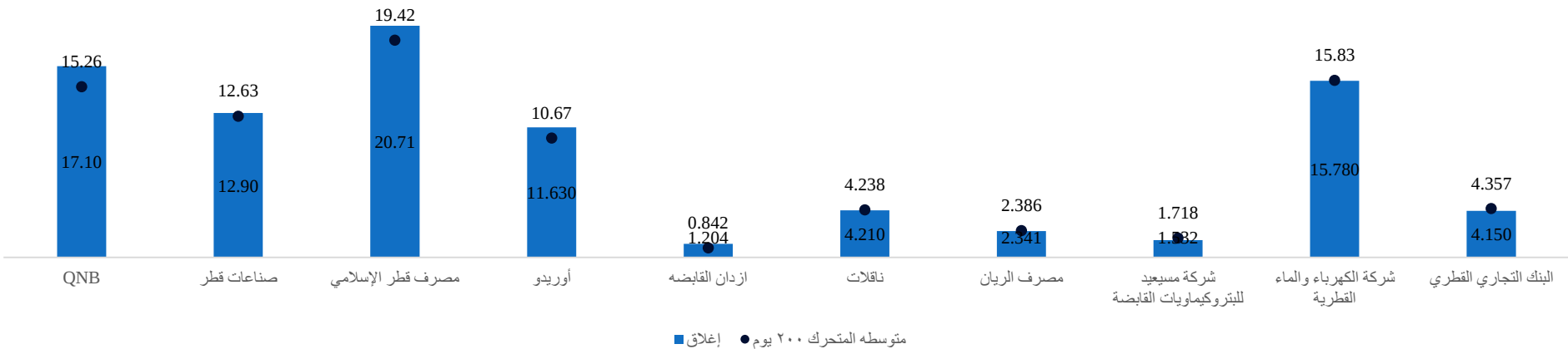
مستوى إغلاق السهم بالمقارنة مع متوسطه السعري المتحرك – ٢٠٠ يوم
